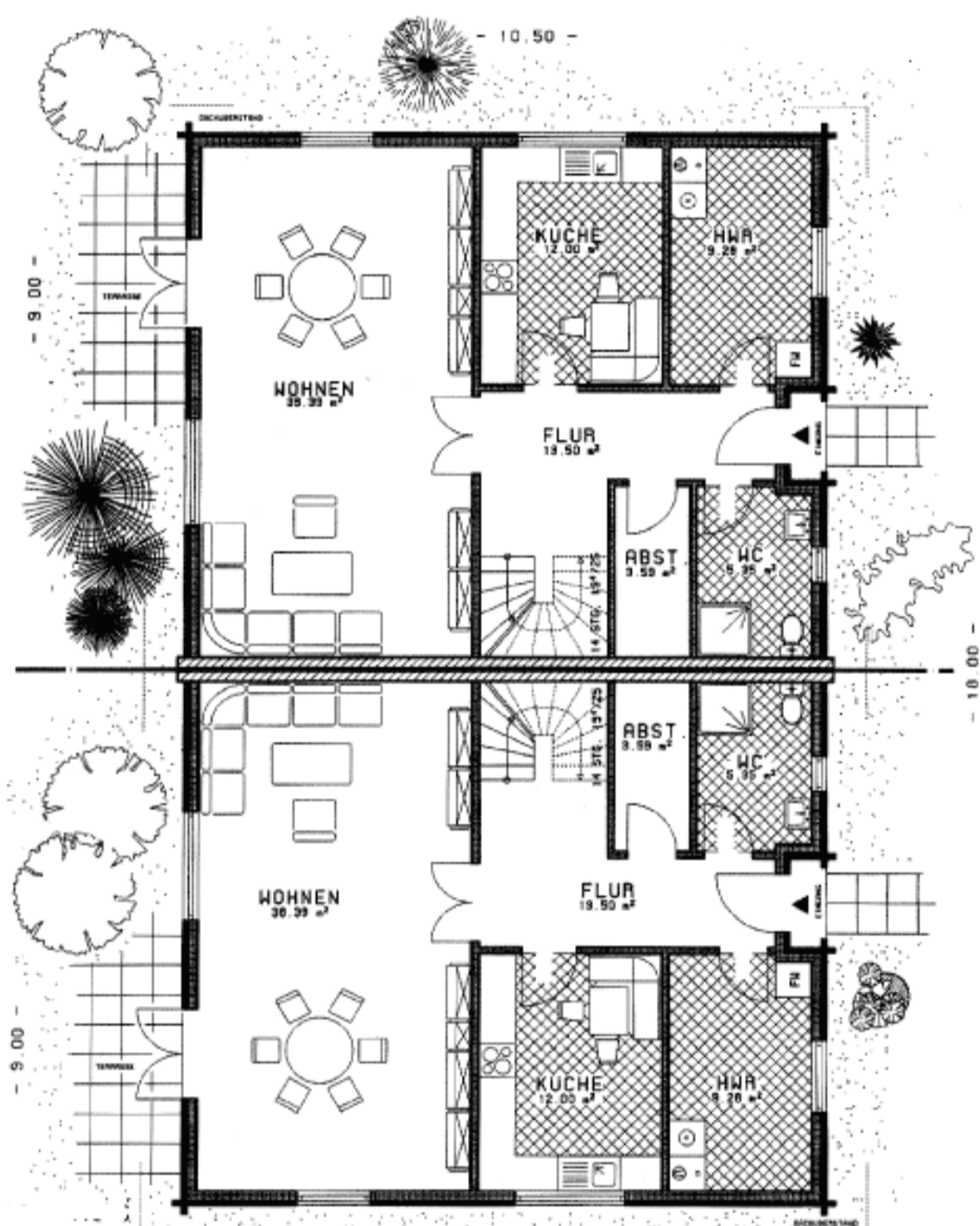
Erdgeschoss
